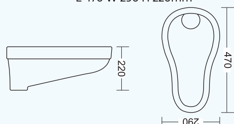
GI-433 | IWC (18\") OPEN RIM
